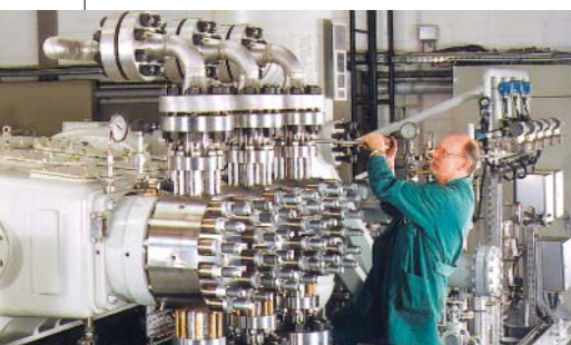
LEWA triplex
