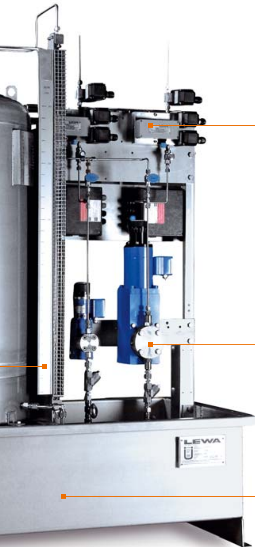
Блок одоризации OD 240
